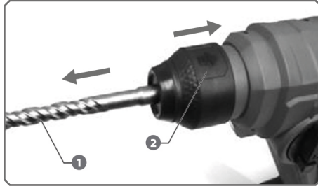
1. Broca de perfuração SDS 2. Cobertura do Mandril
